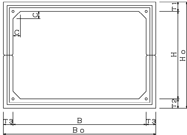
正面図
