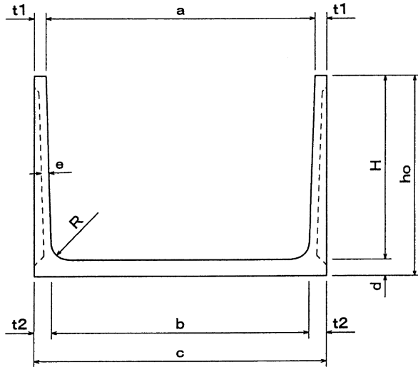
正面図
