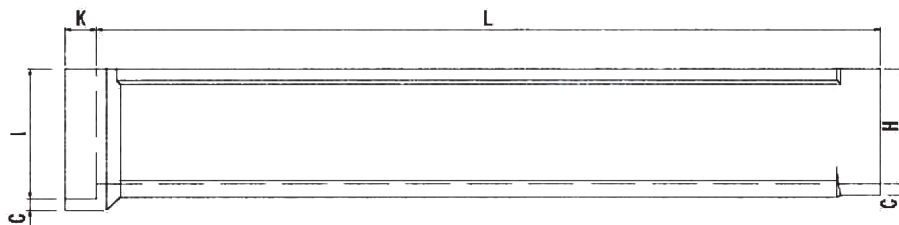
側面図
