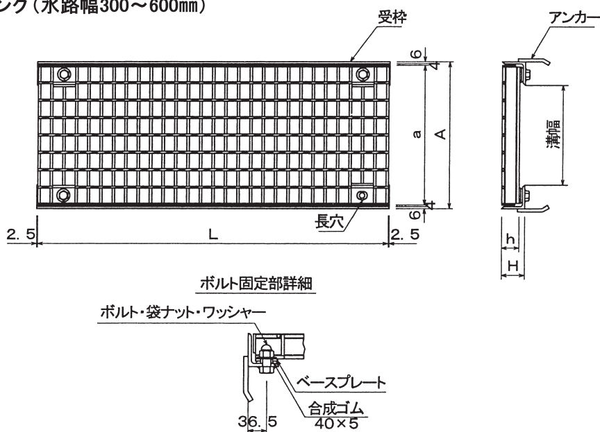
横断用グレーチング(水路幅300~600mm)
