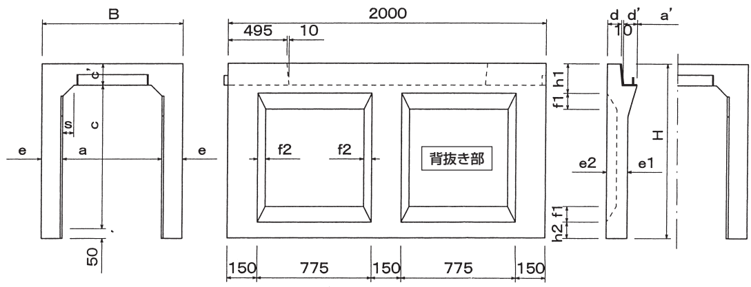
■ 規格図(水路幅700~1000mm)
