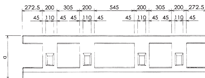
平面図
