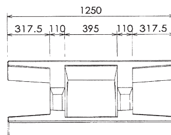
平面図
