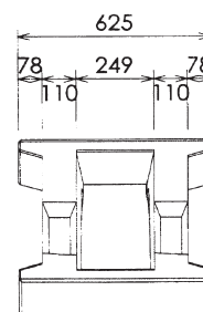
平面図
