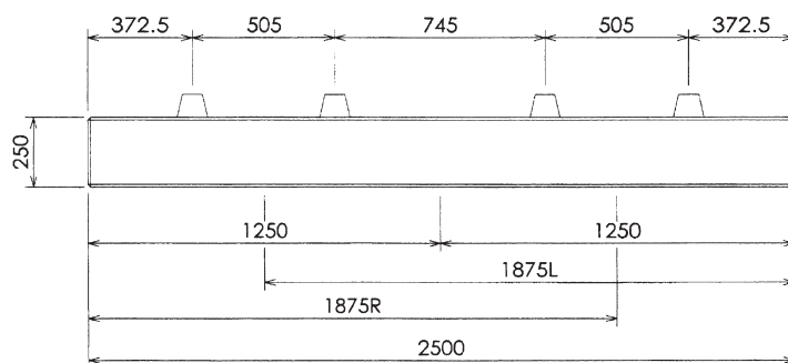
正面図
